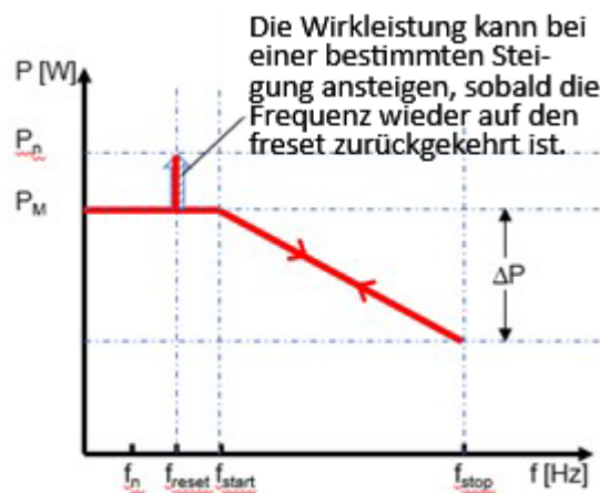
Abb. 71. Ohne Hysterese
