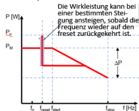
Abb. 72. Mit Hysterese
