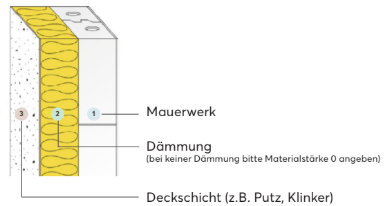
Schnitt Wandaufbau
