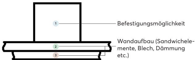
Wandaufbau Draufsicht
