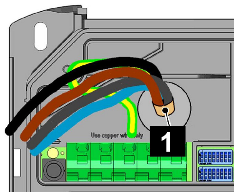
Doppelmembranstützen (Unterputz Kabelmontage)
