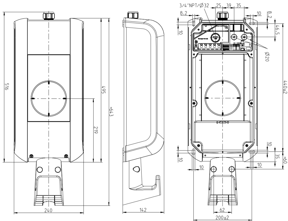
Abb. 12-21: Abmessungen in Millimeter
