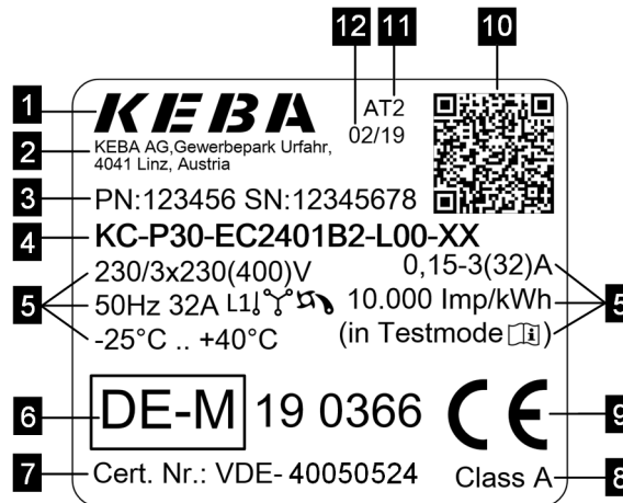
Abb. 4-7: Typenschild (Beispiel)
