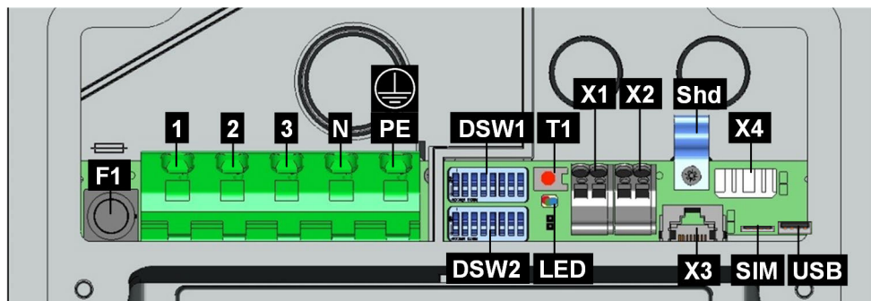
Abb. 7-15: Anschlussübersicht
